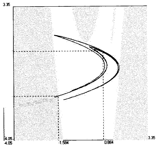
Рис. 9. Неустойчивое многообразие седла системы Хенона. Затемненная часть квадрата — начальные данные, при которых траектории стремятся к бесконечности.
