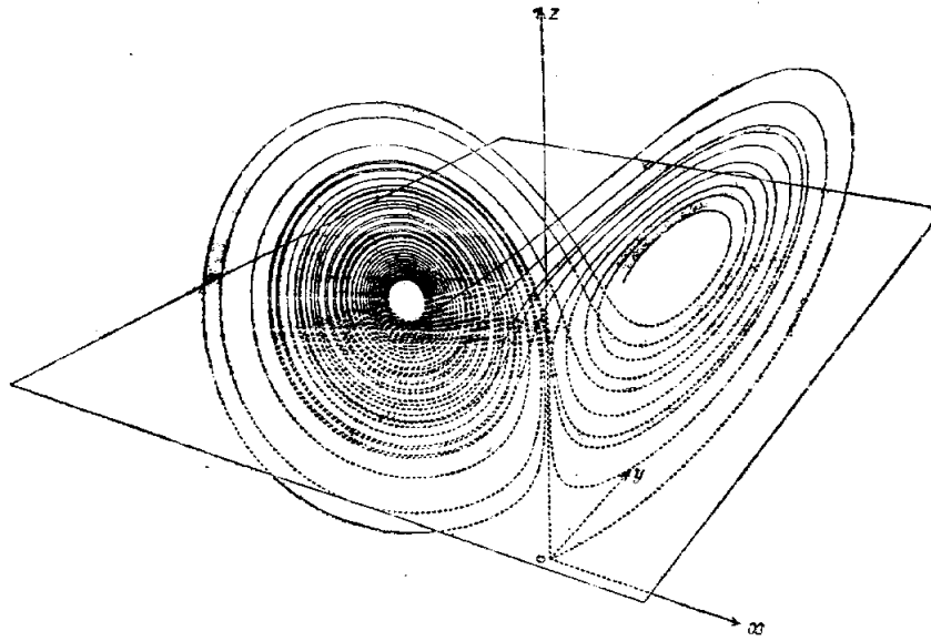
Рис. 7. Неустойчивое многообразие седла системы Лоренца. Первые пятьдесят оборотов.
