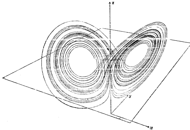
Рис. 8. Неустойчивое многообразие седла системы Лоренца. Следующие пятьдесят оборотов.
