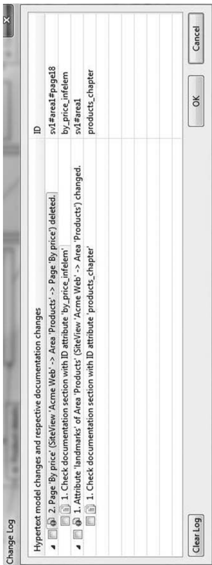
Рис. 5. Журнал изменений
