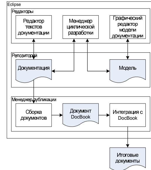
Рис. 13. Архитектура пакета инструментальных средств
