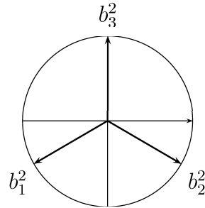
Рис. 4. Фрейм Мерседес-Бенц в пространстве \mathbb{R}^2
